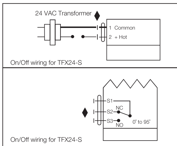
Fig. 5 24 VAC/VDC Actuator
