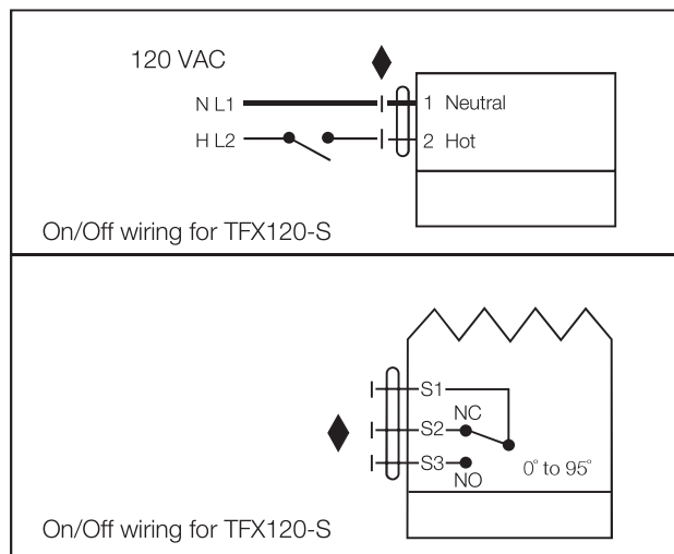
Fig. 4 120 VAC Actuator
